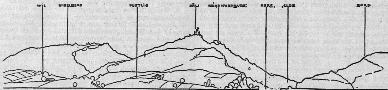
BERGE IM SÜDEN V. OLTEN
