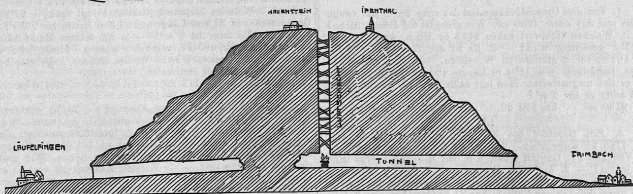
DAS UNGLÜCK BEIM BAU DES HORNSTEINTUNNELS 28. I. 1857
