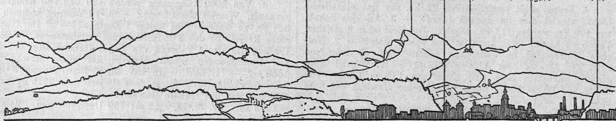
DER JURA IM NORDEN VON OLTEN
