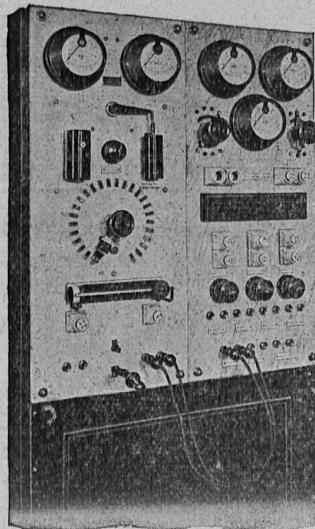
Gleichrichter-Anlage mit Experimen- teller Schalttafel in einem Gymnasium.
