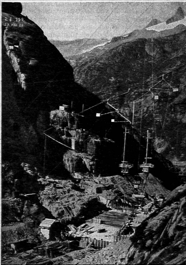
Installationen für die Betonplacierung in der Spitallamm.
