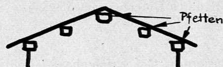
reines Pfettendach
