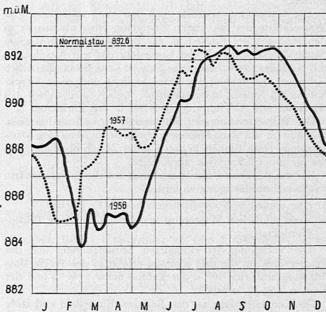
Abb. 4 Wasserstände des Sihlsees in den Jahren 1956 und 1957.
