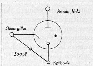
Fig. 3 Kaltkathodenröhre
