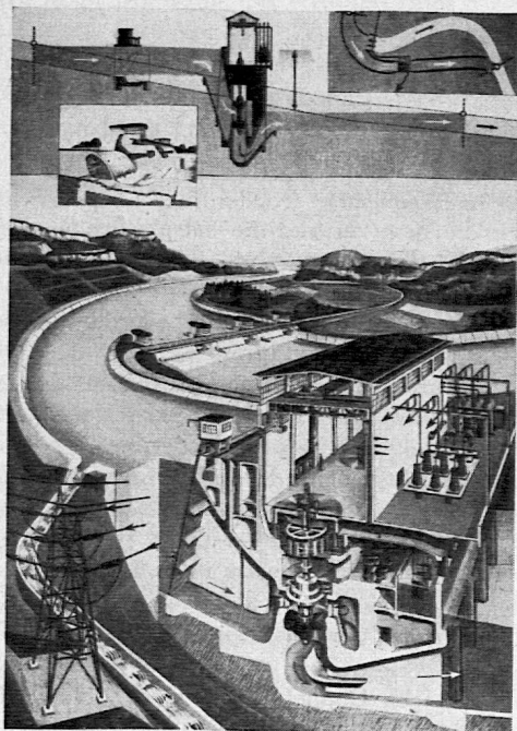
Abb. 2 Niederdruck-Laufwerk
