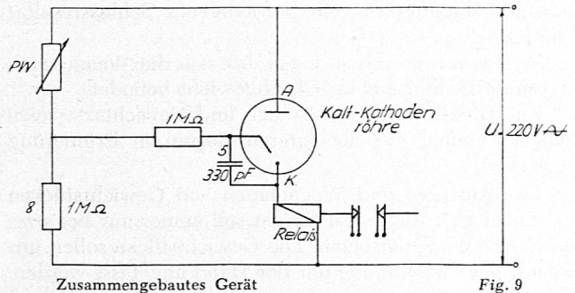
Zusammengebautes Gerät Fig. 9
