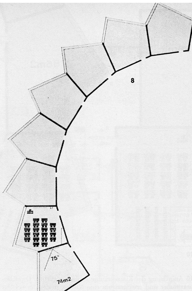
8 Die in der vorhergehenden Abbildung gezeigte Raumform umschliesst, aneinandergefügt, eine im Grundriss kreis-segmentförmige Halle. Dieser Vorschlag weist gegenüber der normalen sägeförmigen Anordnung folgende Vorteile auf:
