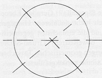
Kreis, axialsymmetrisch in bezug auf jeden Durchmesser
