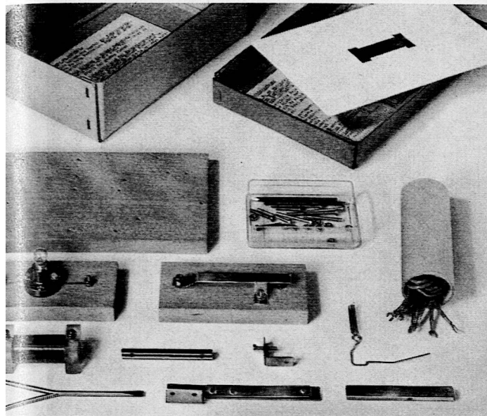
Bausatz B (reihenweise von links oben nach rechts unten): Experimentierbrett, Kleinmaterialschatel mit Zutaten, Lämpchenhalter, Taster/Schalter, Kabel, Spule, Kern, Kontaktwinkel, Zeiger, Schraubenzieher, Summerzusatz, Telegraphenzusatz.
