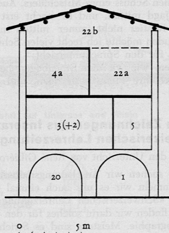
Abb. 5 Brusio. Haus mit übereinanderliegenden Oekonomie- und Wohnräumen. Schematischer Querschnitt. Unterstes Geschoss: gewölbter Stall und gewölbter Keller; zweites Geschoss: Stube und Küche, an einem Korridor liegend; drittes Geschoss: Heustall mit abgegrenztem Bezirk für das Lager des Vaters und der Knaben. (Die Mutter verblieb mit den übrigen Kindern in der Stube.) Die obersten Fensterchen dienen der Lüftung. In ihrer Höhe hängen die Garben. Hier auf dem Dachboden wurde der Buchweizen gedroschen.
