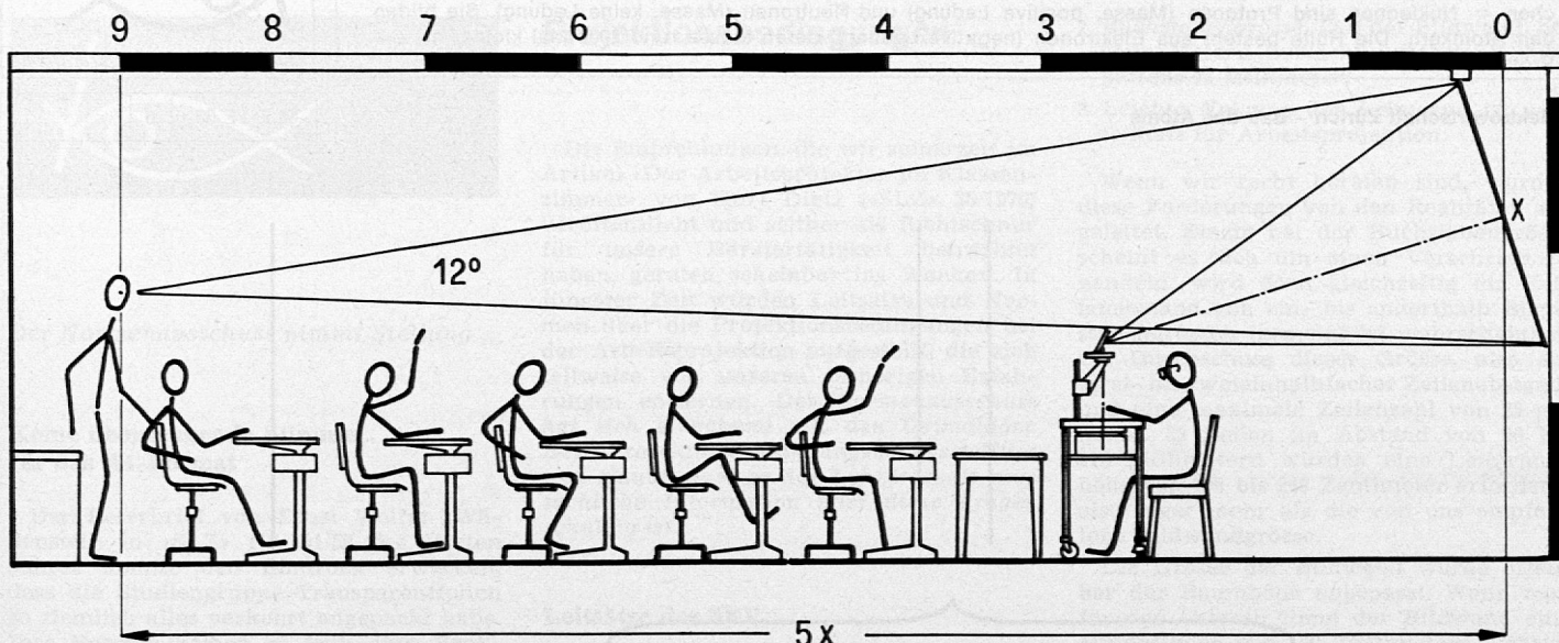
Bild 2 – Mindestanforderungen für die Bildprojektion
