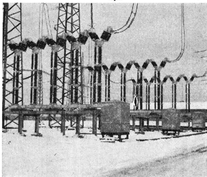
Ölarmer Leistungsschalter Typ HPF 516 in Kilforsen, Schweden
