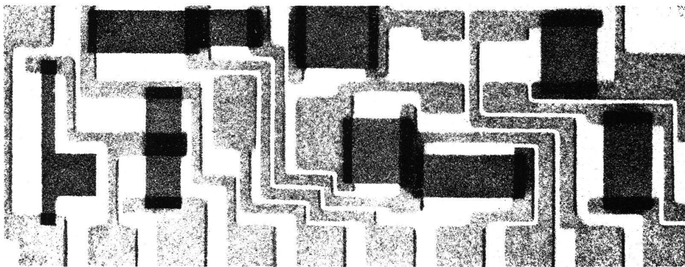
Dickfilmschaltung / Ausschnitt
