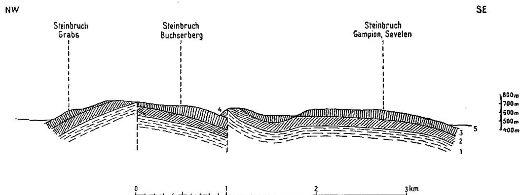
Fig. 4. Querprofil durch das Rheintalvorkommen. 1 = Drusbergsschichten, 2 = oberer Schrattenkalk, 3 = mittlere Kreide, 4 = Seewerkalk, 5 = Alluvium.
