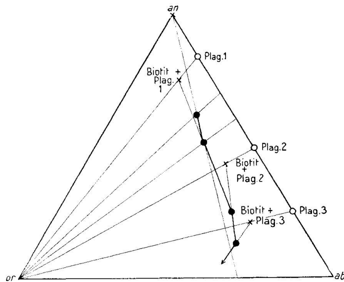
Fig. 25. Schematischer Verlauf der Kristallisationsbahn bei längerer Zeit gleichartiger Ausscheidung von Gemengen von Plagioklas + Biotit.
