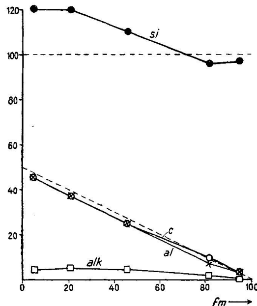
Fig. 1. Differentiationsdiagramm der Hauptgesteine der kritischen Zone. Mit sinkendem fm -Gehalt steigen c und al linear an; alk bleibt immer niedrig, si ändert sich wenig. Die gestrichelt gezeichnete, schräg verlaufende Linie wäre der Ort der Projektionspunkte von al und c , einer einfachen Variation Anorthit-Orthaugit. In diesem Falle müsste si konstant = 100 sein.
