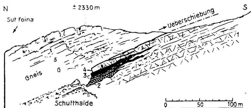
Fig. 1. Profilansicht der Eisen - Manganerzlagertstätte Fianell I (nach (5), etwas abgeändert).
