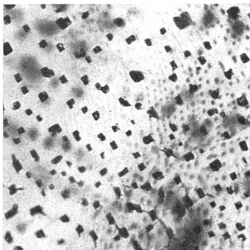
Fig. 3. Reihen euhedraaler Spinell-Oktäeder in Spinell aus Burma, 150 \times
