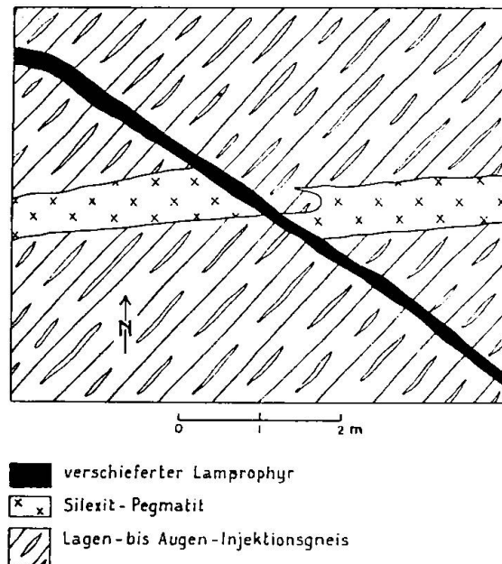
Fig. 2. Gangkreuzung. E-Abhang des Rossbodenstockes. Grundriss. Silixitpegmatit durchbricht Lagen- bis Augen-Injektionsgneis und wird seinerseits diskordant von verschieferem Lamprophyr durchbrochen, der längs einer Verwerfungsspalte eingedrungen ist. Der Silixitpegmatit ist an der Verwerfung verstellt. Siehe auch Fig. 1 der Tafel II.
