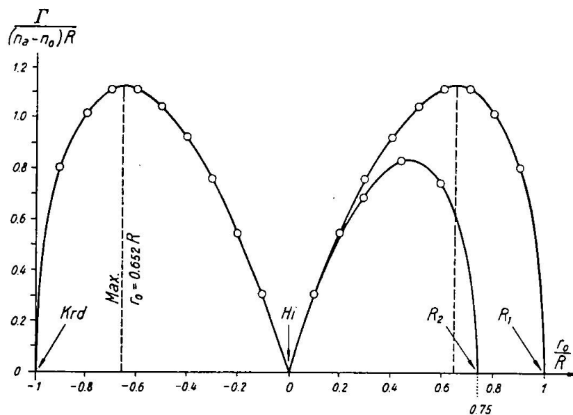
Fig. 1. Gangunterschied I' eines Sphäriten in Funktion von r_0 ( r_0 = Abstand vom Sphäritenzentrum, H_i = Hilum, Krd = Kornrand). Rechts: Der Gangunterschied einer Hohlkugel vom Radius R_1 = 1 und einem Hohlraum vom Radius R_2 = 0,75 ist gegeben durch die Differenz der beiden angegebenen Kurven; vgl. Formel (3)
