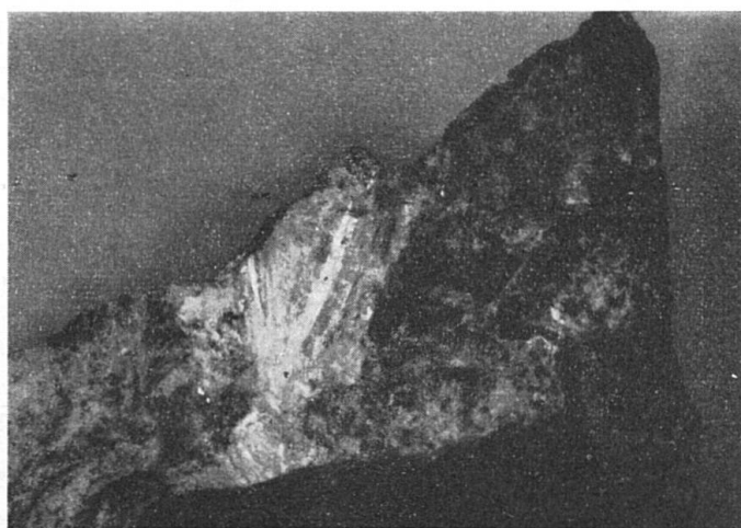
Fig. 1. Linealartige Kristalle von Brandtit bilden ein strahliges Aggregat in einer Zerrklüft im Brauniterz (schwarz). \frac{4}{5} nat. Grösse
