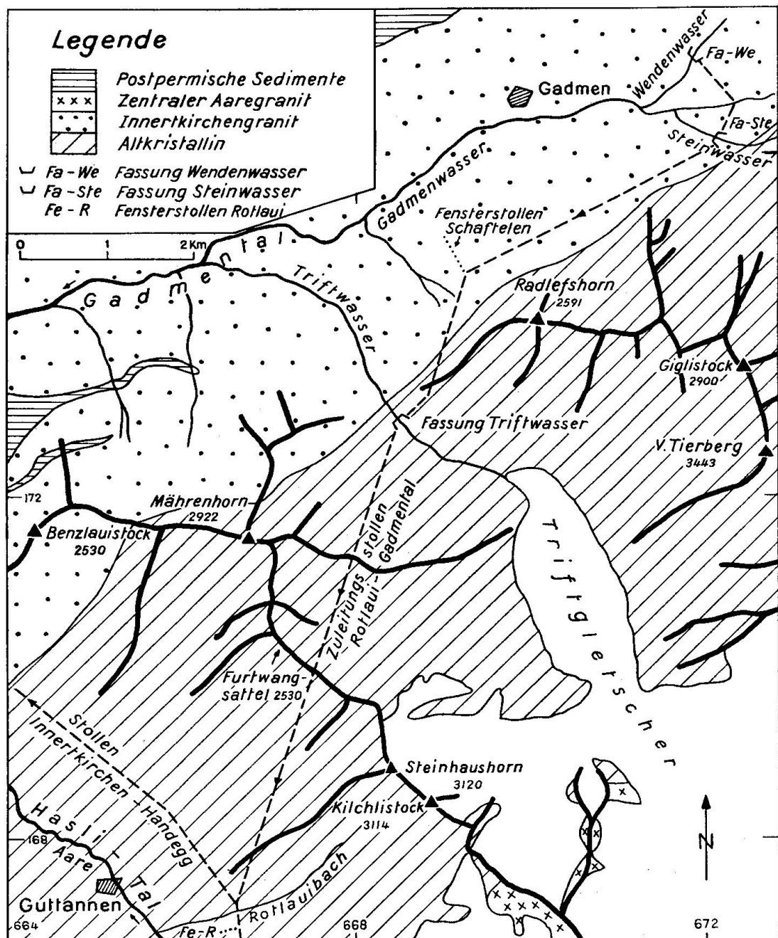
Fig. 1. Lageskizze des Zuleitungsstollens Gadmental-Rotlauri (Haslital) der Kraftwerke Oberhasli AG (Aarmassiv). 1 : 75 000.
