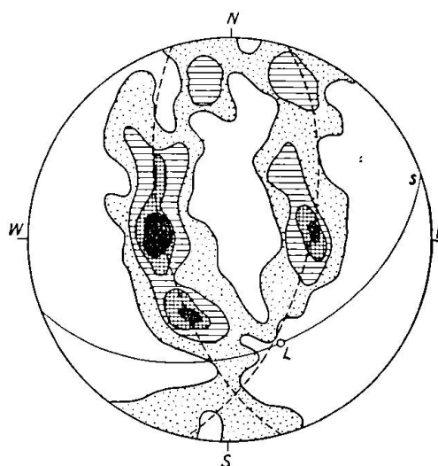
Fig. 22. Quarz. 1000 c-Achsen. 1, 2, 3, 4%. Max. 4,5%. Horizontalschliff. Quarzit, Frodamera, Pioramulde.
