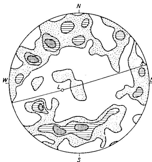
Fig. 21. Quarz. 300 c-Achsen. 1, 2, 3%. Max. 3\frac{1}{3}\% . Schliff 6^\circ gegen N geneigt. Sandkalk, Pardatsch, Val Nalps, Urseren-Garvera-Mulde.
