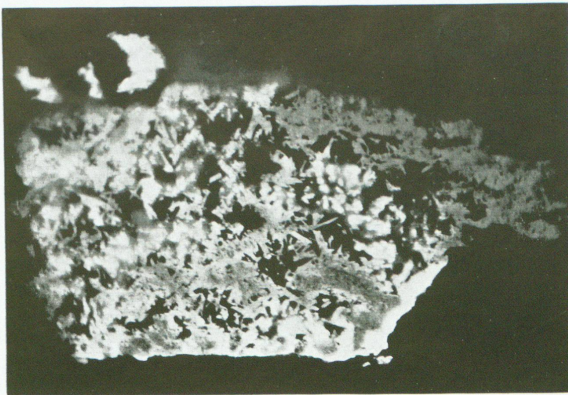
Abb. 1. Rutil und Anatas (weiss) sind umkrustet von Brannerit, zum Teil sehr schön nadelig (hell-dunkelgrau). Gesteinsgrundmasse schwarz. 1 Nicol, Ölimmersion, Vergr. ca. 500 \times . Mürtschenalp.
