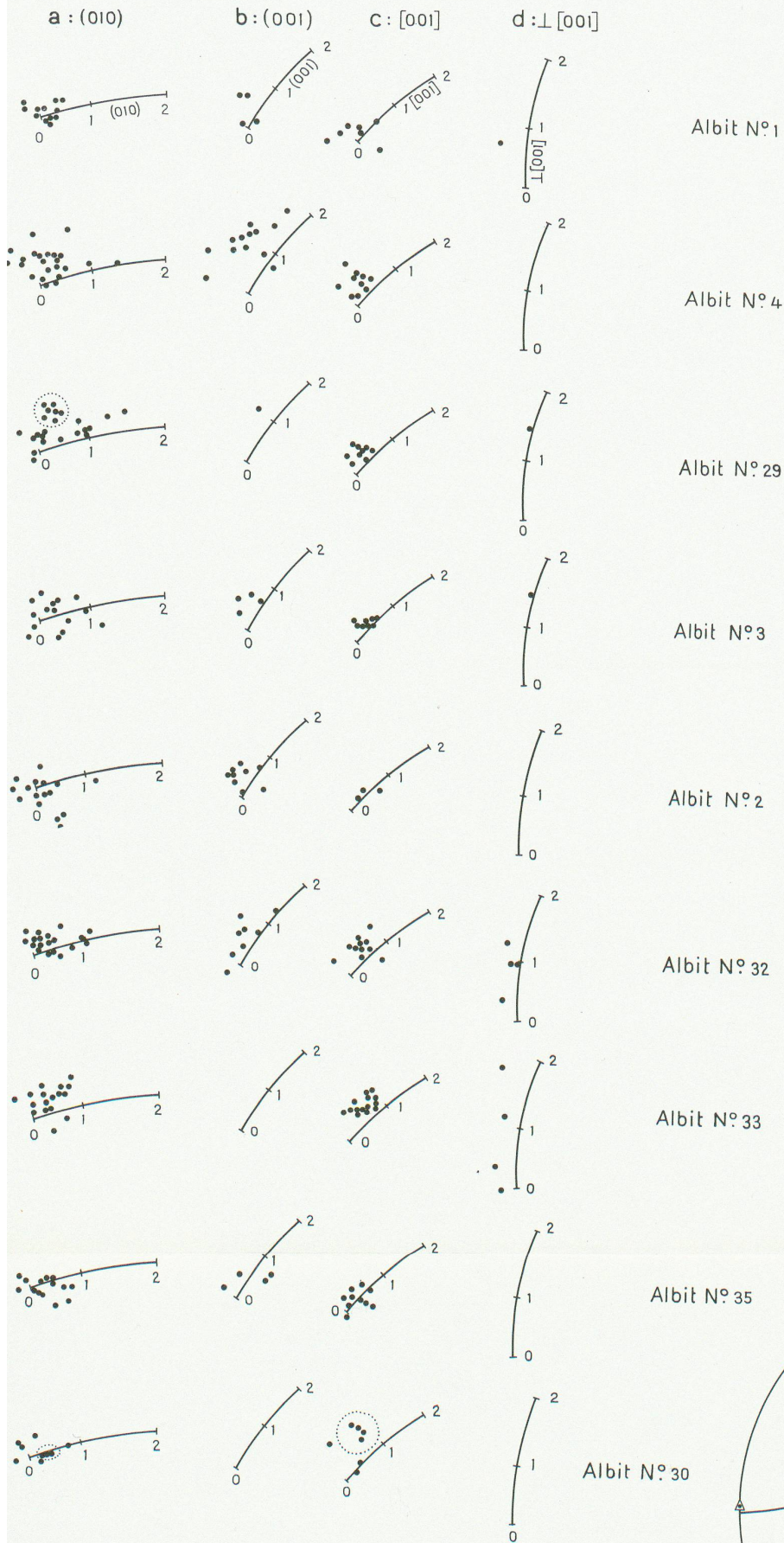
Lage der Kurventeile a-d auf dem Stereogramm \perp n\beta
