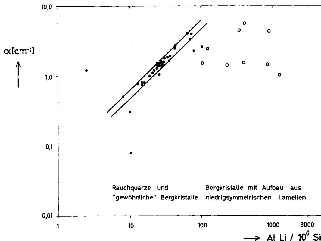
Fig. 7. Zusammenhang zwischen Extinktionskoeffizient \alpha [cm -1 ] ( n_{\omega}, 466 \text{ m}\mu ) \gamma -bestrahlter Quarze und den aus der Analyse kombinierbaren AlLi-Defekten. ● gewöhnliche Quarze, ○ Bergkristalle mit Aufbau aus niedrigsymmetrischen Lamellen, × die Bergkristalle Q 309, Q 310 mit [\text{H}] > [\text{Li} + \text{Na}] . Darstellung im log-Massstab.
