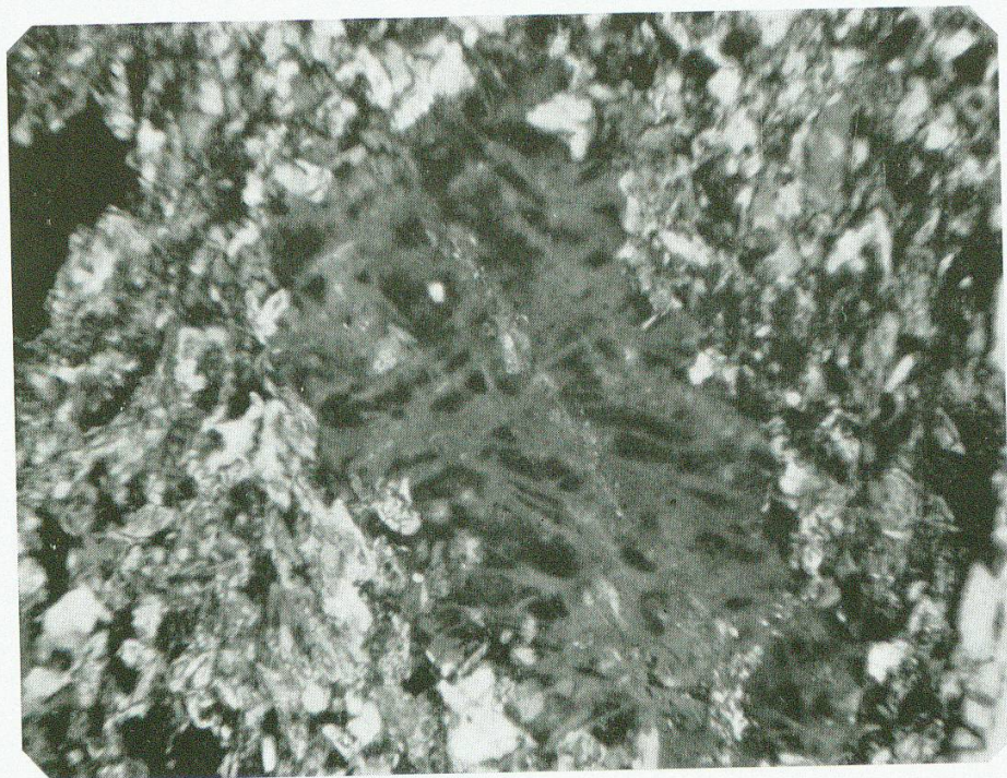
Photo n° 7. Feldspath potassique à taches sombres. Echantillon Roffna n° 5. G = 28 \times . Nicols croisés.
