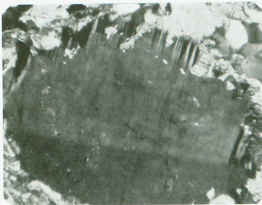
Photo n° 9. Plage de feldspath potassique maelé selon Manebach, avec macles lamellaires selon l'albite à la périphérie. Echantillon Roffna n° 7. G = 100 ×. Nicols croisés.
