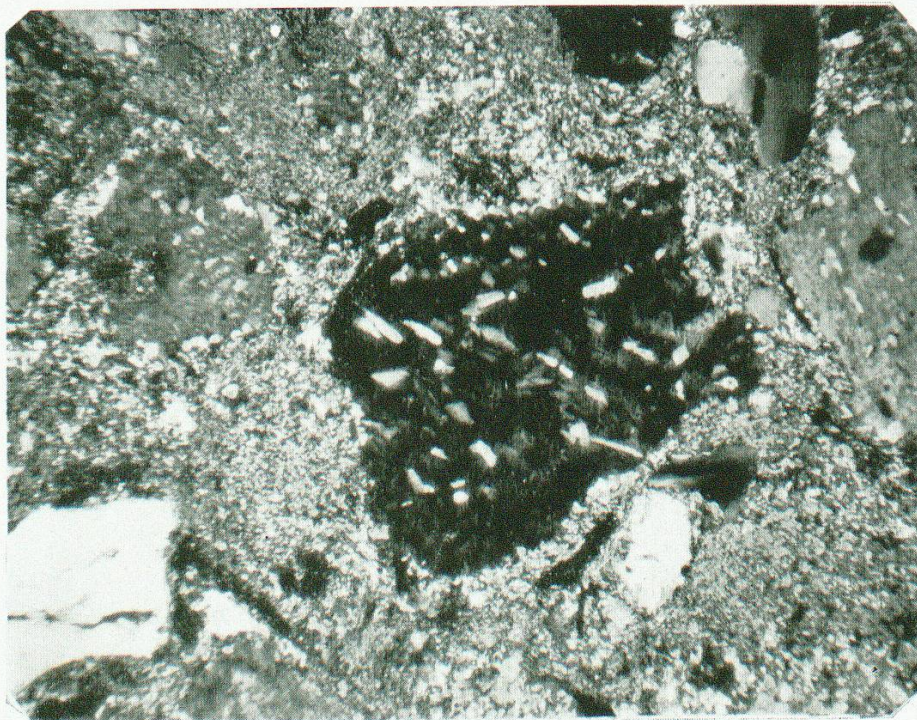
Photo n° 4. Pâte quartzo-feldspathique séricitique cimentant des fragments de quartz et de feldspath potassique à inclusions microlitiques d'albite. Echantillon Roffna n° 2. G = 20 \times . Nicols croisés.
