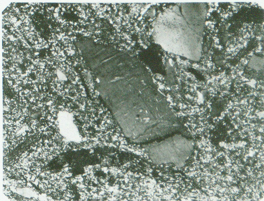
Photo n° 11. Fragment de feldspath potassique à lames d'albite. Echantillon Roffna n° 8.
