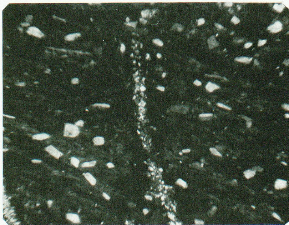
Photo n° 2. Inclusions microlitiques d'albite dans le feldspath potassique. Echantillon Roffna n° 1. G = 80 \times . Nicols croisés.
