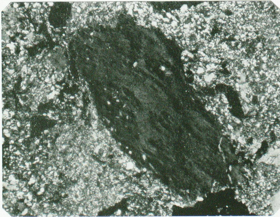
Photo n° 3. Feldspath potassique à marbrures sombres. Echantillon Roffna n° 1. G = 32 \times . Nicols croisés.
