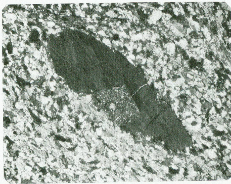
Photo n° 8. Fragment lenticulaire de feldspath potassique à inclusions rectangulaires de plagioclase séricitisé. Ech. Roffna n° 7. G = 45 \times . Nicols croisés.
