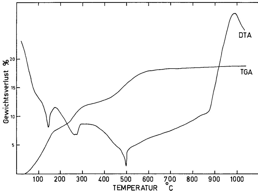
Fig. 2. DTA- und TGA-Kurven von Palygorskit aus dem Entlebuch. Aufheizgeschwindigkeiten: DTA 9,5^{\circ}\text{C} pro Minute, TGA 2,5^{\circ}\text{C} pro Minute.
