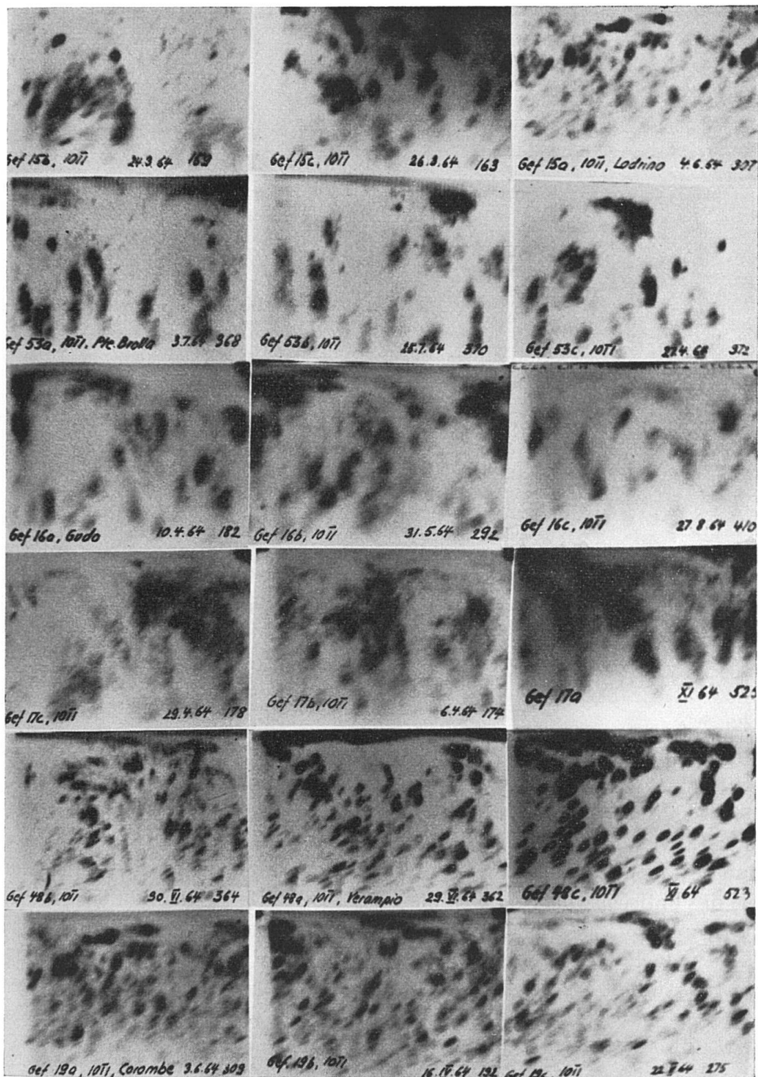
Fig. 49. Röntgendiagramme von Überindividuengefügen. Verteilung der Netzebene (1011). Charakteristisch sind die zahlreichen starken Einzelmaxima und die niedrige Symmetrie. Von jeder Probe wurden drei senkrecht zueinander stehende Schnitte aufgenommen. Die erste Kolonne enthält Diagramme von ac-, die zweite von be- und die dritte von ab-Schnitten (nähere Erläuterungen siehe Text).
