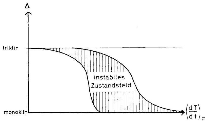
Fig. 2. Schematische Darstellung der Triklinitätsverteilung von Feldspäten in metamorphen Gesteinen als Funktion der Abkühlungsgeschwindigkeit. ( \Delta = Triklinität, dT/dt = Abkühlungsgeschwindigkeit.)
