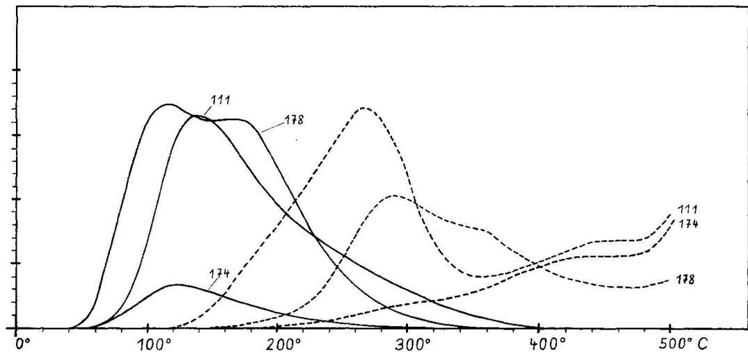
Fig. 2. Die Glow-Kurven der natürlichen und durch Röntgenstrahlung erzeugten Thermolumineszenz am Beispiel des Albites von Portland (Nr. 178) und der Oligoklasse von Bakersville (Nr. 111) und Hemet (Nr. 174). Die Intensitäten der natürlichen Thermolumineszenz verhalten sich zur künstlichen bei den Proben Nr. 111 und 174 wie 1 : 500, bei 178 wie 1 : 200.
