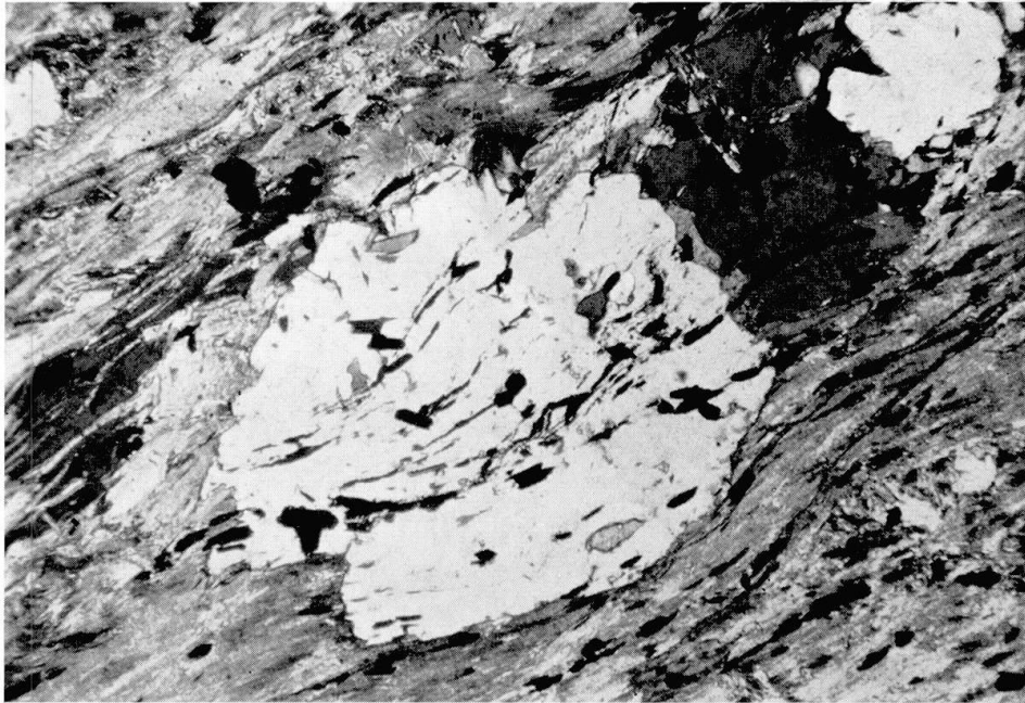
Fig. 3. Phyllite chlorito-séricitique en voie d'albitisation. Porphyroblaste d'albite avec inclusions alignées d'oxydes de fer. Lumière polarisée. Ech. n° 105. G = 30 \times .
