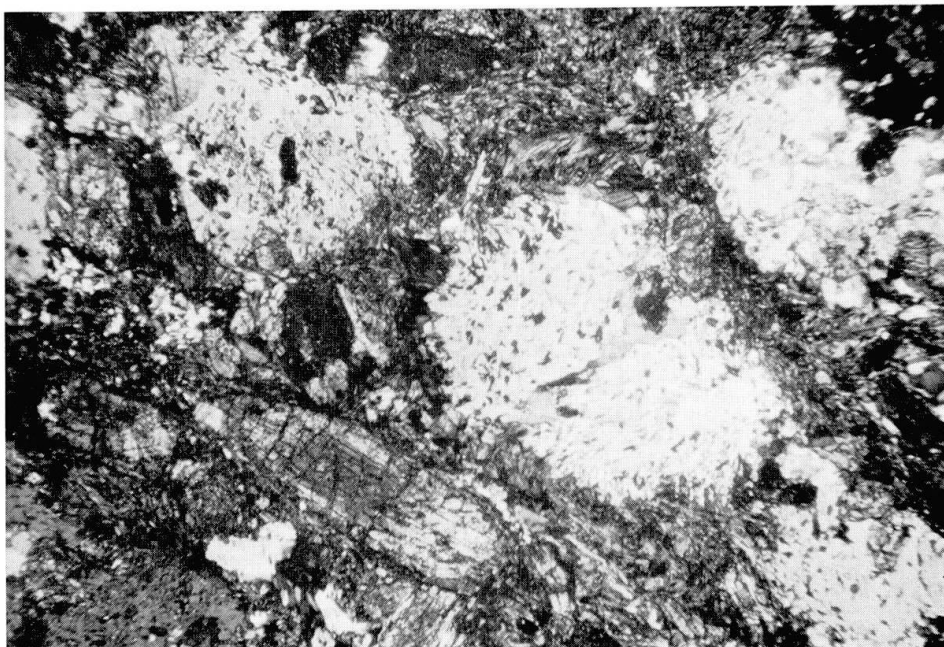
Fig. 2. Prasinite à hornblende n° 187. Lumière polarisée. G = 20 \times .
