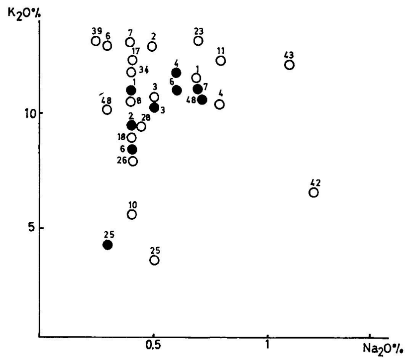
Fig. 11. Kalium- und Natriumgehalte der hellen Glimmer. ○ Nebengesteinsmuskowite, ● Kluftmuskowite.
