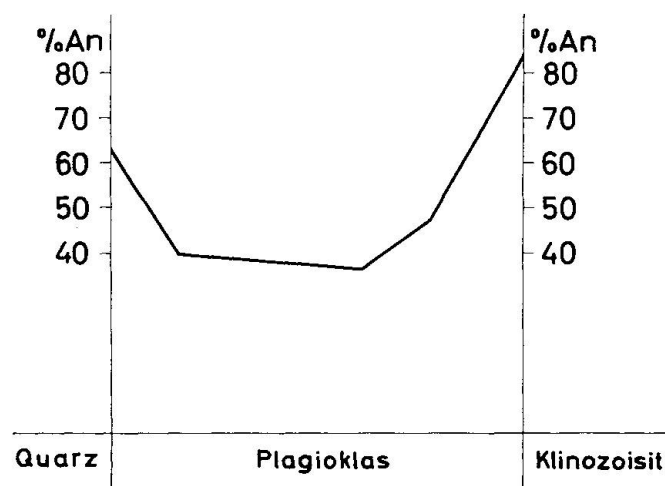
Fig. 8. Einfluss von Klnzoisit-Epidot auf den Anorthitgehalt von Plagioklas in Amphiboliten. Punktiert: Amphibolite ohne Epidot. Schwarz: Amphibolite mit Epidot. Die Messungen beziehen sich entweder auf Lagen derselben Probe, oder auf Proben vom gleichen Fundort.
