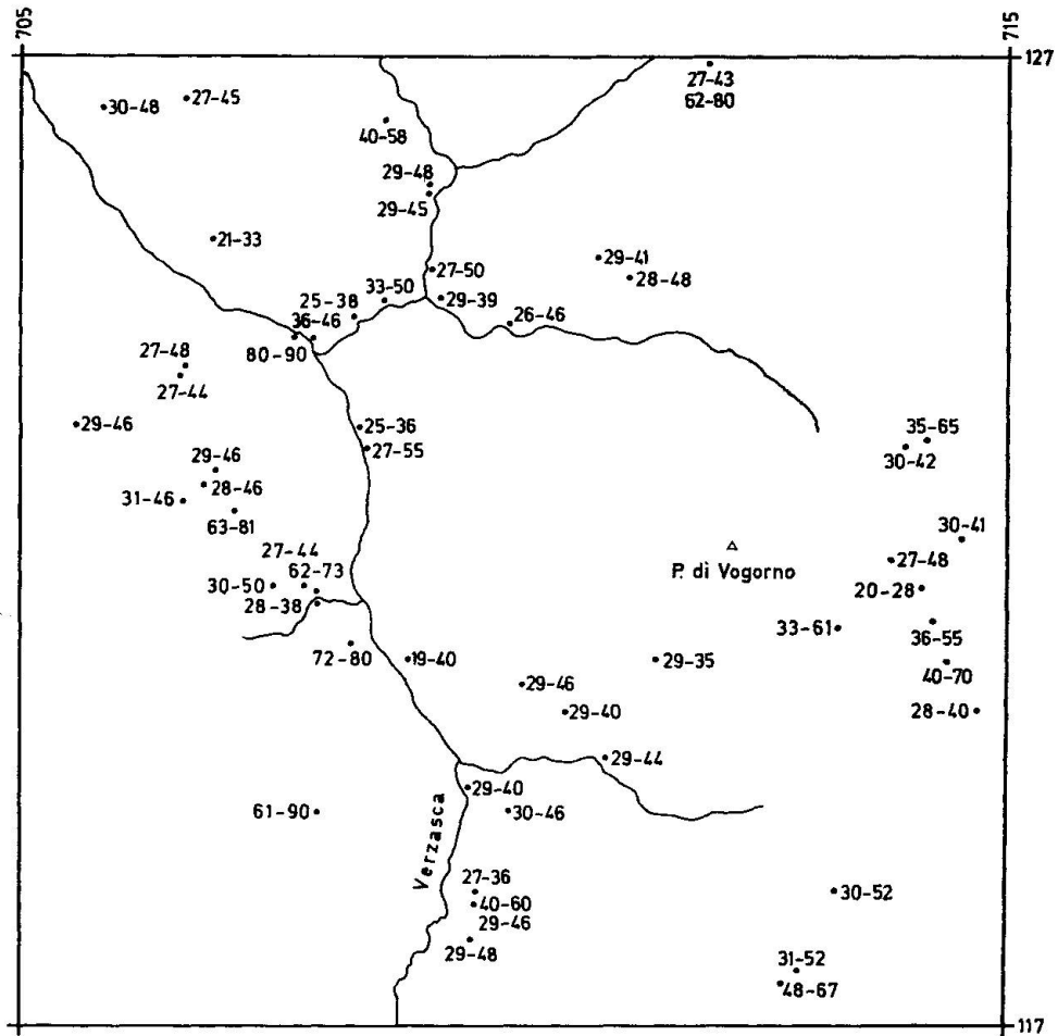
Fig. 1. Verteilung der modalen Anorthitwerte von Amphiboliten im südlichen Teil des Verzasca-tales (P. di Vogorno). Die Kantenlänge des Quadrates beträgt 10 km (Koordinaten 117 bis 127, 705 bis 715).
