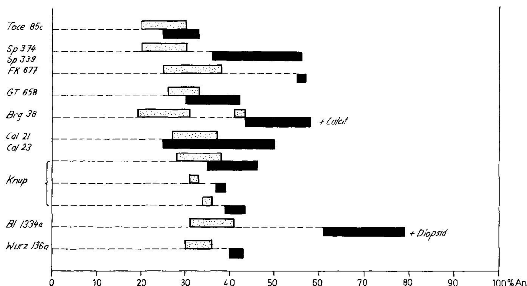
Fig. 8. Einfluss von Klnzoisit-Epidot auf den Anorthitgehalt von Plagioklas in Amphiboliten. Punktiert: Amphibolite ohne Epidot. Schwarz: Amphibolite mit Epidot. Die Messungen beziehen sich entweder auf Lagen derselben Probe, oder auf Proben vom gleichen Fundort.
