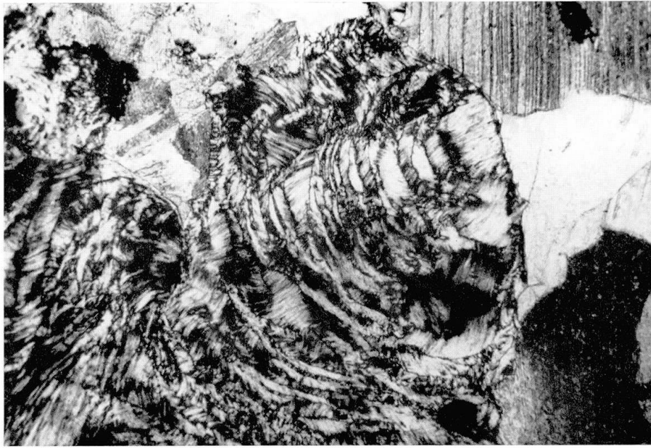
Fig. 2. Konzentrische Deformationsbänder in Brucit. Rechts (hell) ein Dolomittkorn, oberhalb und unterhalb davon Calcit. + Nicols 28\times .
