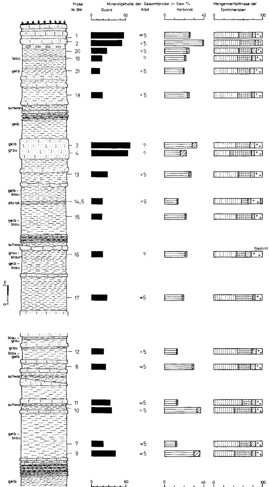
Fig. 3. Schematisches Profil und Zusammensetzung der untersuchten tortonischen Molassegesteine (Bodensee-Schüttung) der Grube Bruggwald/St. Gallen. Legende zum Profil siehe Fig. 1.
