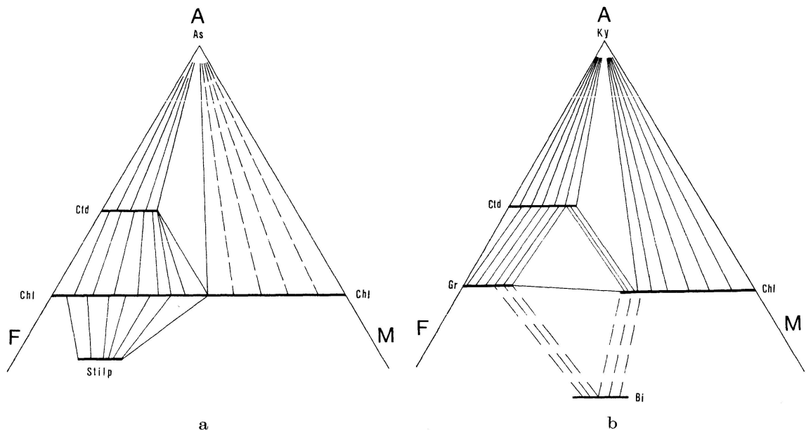
Fig. 6. Phasenbeziehung pelitischer Gesteine in der AFM-Projektion nach THOMPSON. As: Alumosilikat (Pyrophyllit, Disthen), Ky: Disthen, Cld: Chloritoid, Chl: Chlorit, Gr: Granat. Erklärung im Text.
