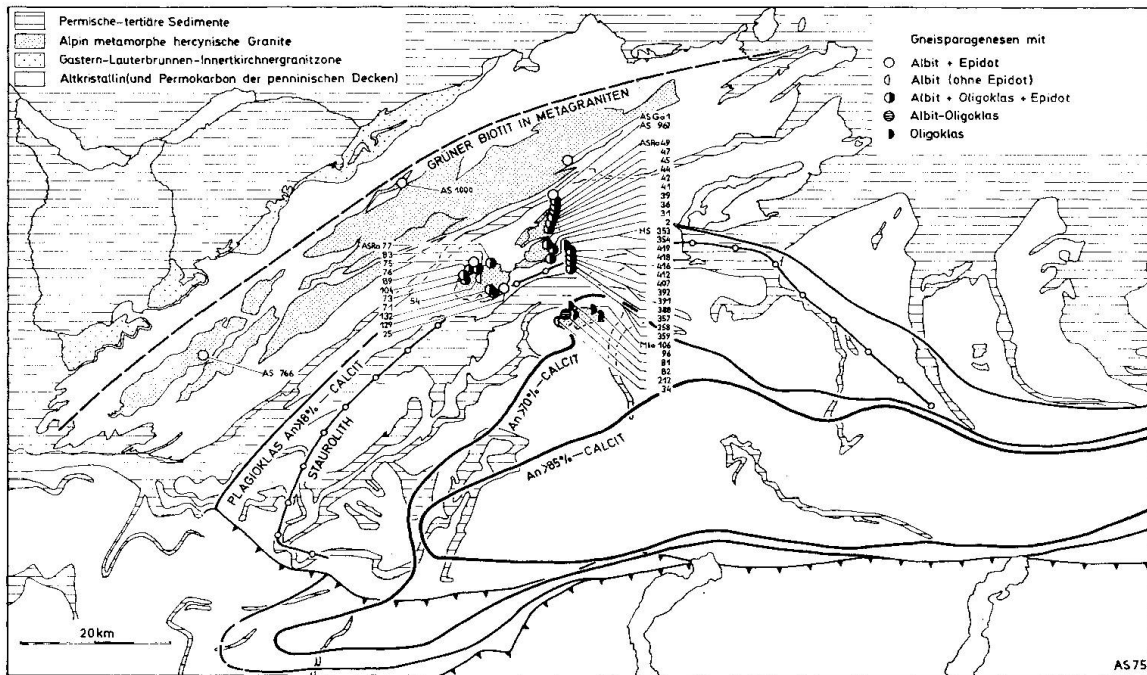
Fig. 1. Fundortkarte der in der vorliegenden Arbeit untersuchten Gneissproben, mit Mineralzonenengrenzen für Biotit in Granitgneisen nach STECK und BURRI (1971), für Staurolith nach E. NIGGLI und C. NIGGLI (1965) und für Plagioklas in Calcitparagenesen nach Wenk (1962).
