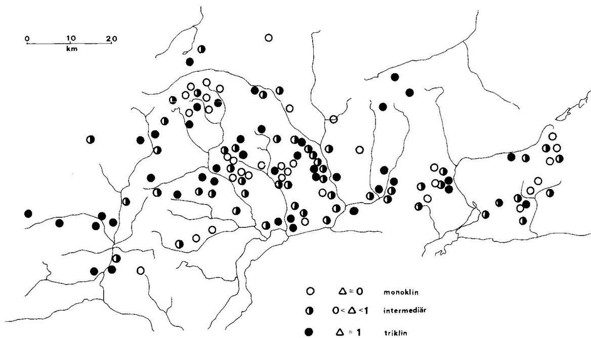
Figur 17: Triaxialitäten der Alkalifeldspäte im Lepontin und angrenzenden Regionen. Intermediäre Triaxialitäten besitzen meist Werte von \Delta \geq 0.75 . Eigene Daten und Daten von Gyr, Hänni und Wenk (op. cit.)
