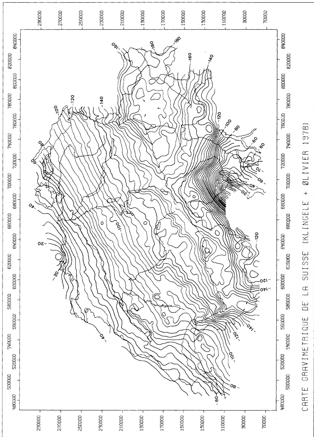
Fig. 1b Gravimetric map of Switzerland (KLINGELE & ØLIVIER 1978).
