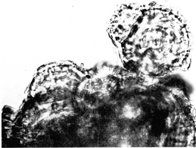
Abb. 2 Arsenocrandallitsphärolithe mit deutlich sichtbarem konzentrisch-schaligem Bau eingebettet in Kanadabalsam. Neubulach. Vergr. ca. 850 x.
