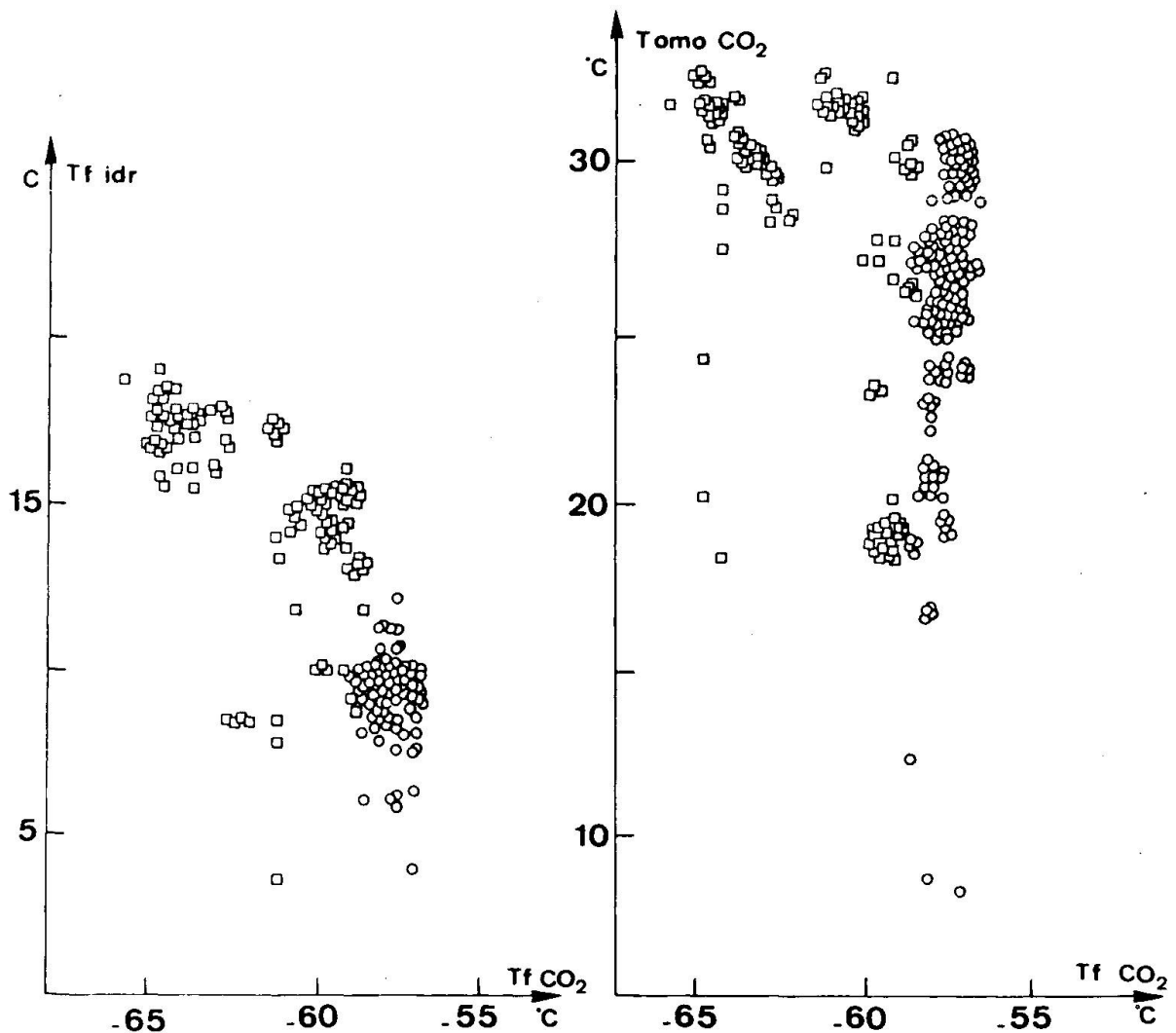
Fig. 20 Diagrammi Tf CO 2 - Tf idr. CO 2 (a) e Tf CO 2 - Tomo CO 2 (b) per le inclusioni a CO 2 puro (circolini) e a CO 2 inquinato (quadratini).
