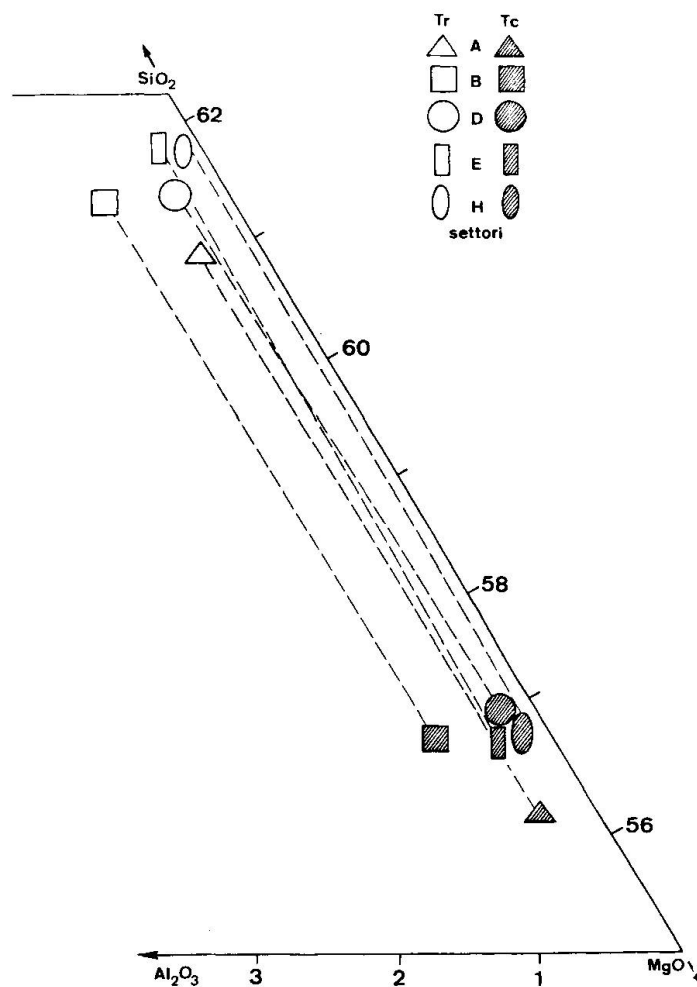
Fig. 11 Distribuzione dell'alluminio tra talco e tremolite in un diagramma SiO 2 -MgO-Al 2 O 3 (Mol %).
