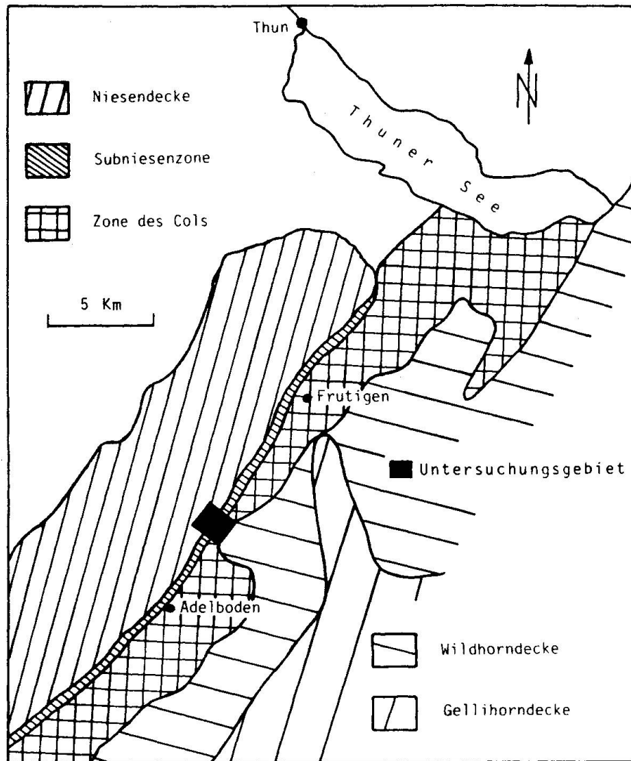
Abb. 1 Regional-tektonische Übersichtskarte.
