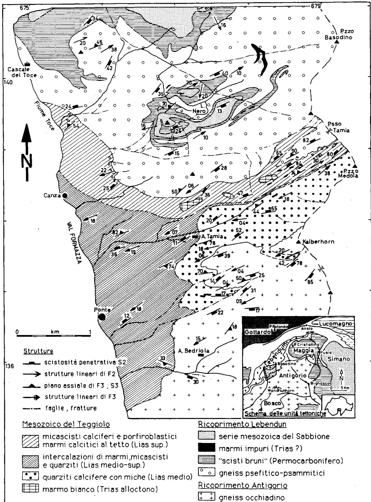
Fig. 1 Carta geologica dell'area considerata.
