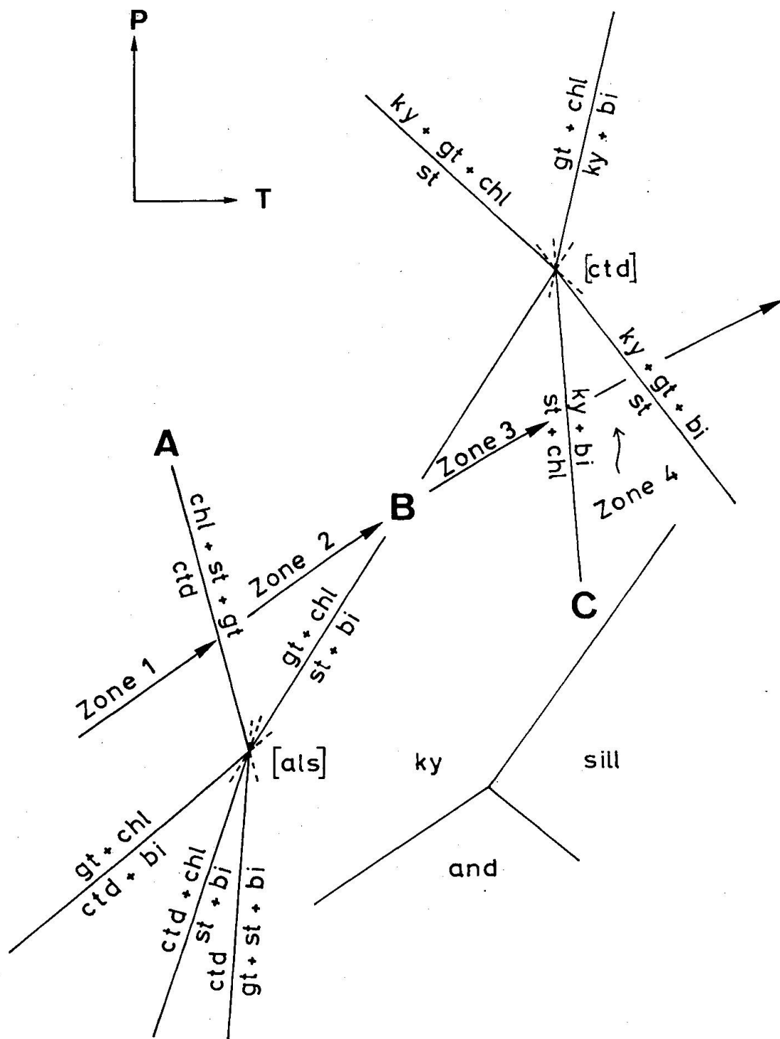
Abb. 4 P-T-Diagramm der Isograd-definierenden Mineralreaktionen in Metapeliten. Gegeben ist der von den untersuchten Gesteinen beschrittene Metamorphoseweg (Zone 1-4).
