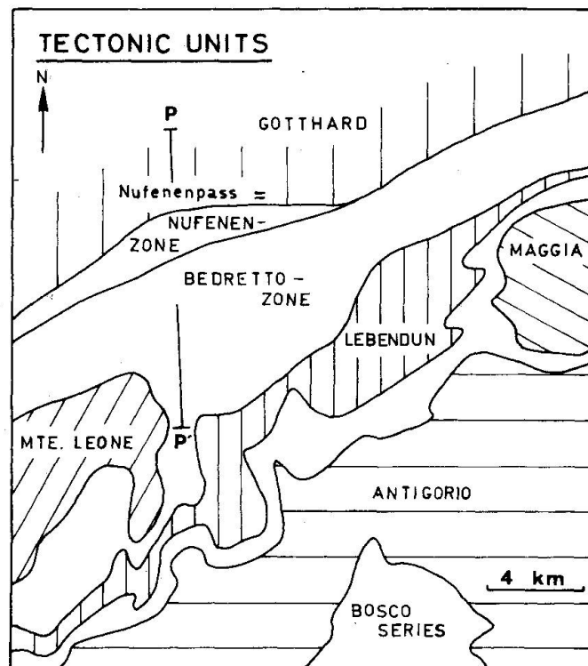
Abb. 1 Tektonische Karte des südlichen Gotthardmassivs und des nördlichen Lepontins (penninische Alpen) im Gebiet des Nufenenpasses (PP': untersuchtes Profil).
