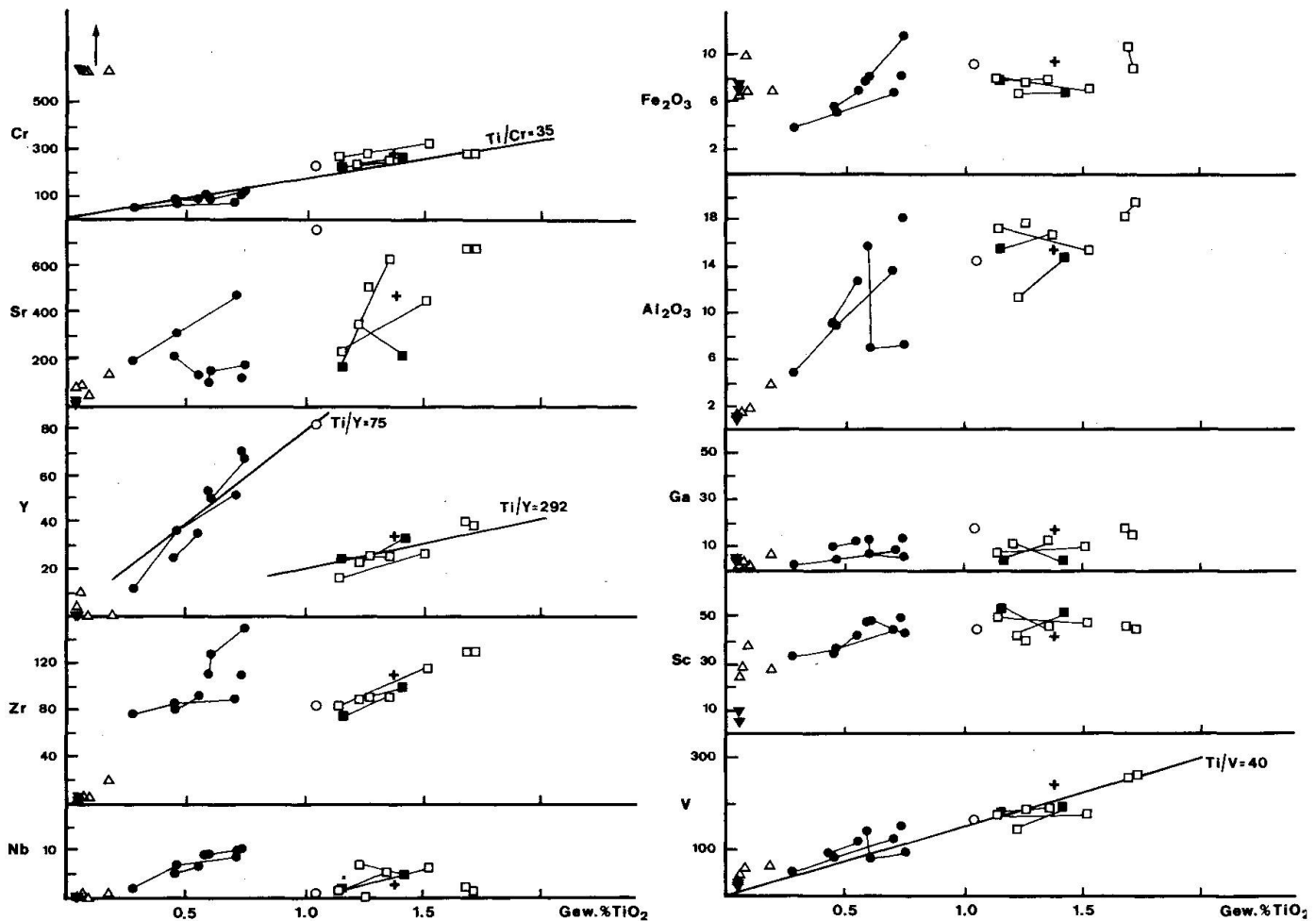
Abb. 3 Variationsdiagramm der Gesteinschemismen versus \text{TiO}_2 . Gesamt-Fe als \text{Fe}_2\text{O}_3 , \text{FeO} , \text{Al}_2\text{O}_3 und \text{TiO}_2 in Gew.%, alle übrigen Elemente in ppm. Legende siehe Abb. 2. Zusätzlich wurden einige Linien gleicher Verteilungskoeffizienten eingezeichnet.
