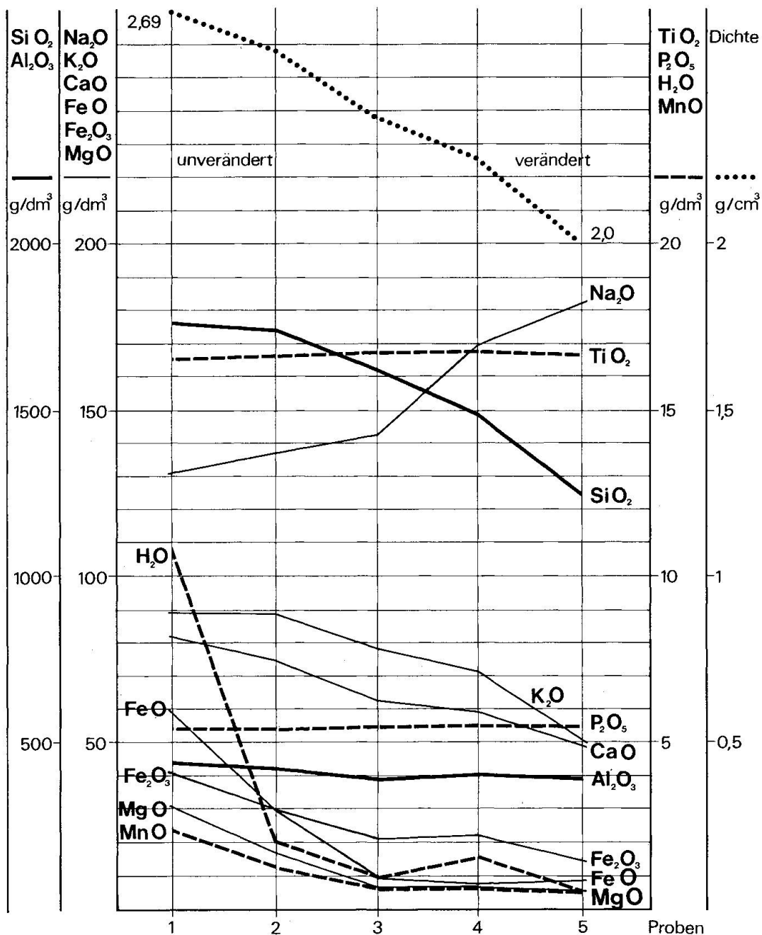
Abb. 1 Geschützte Mineralkluft, Gerstenegg-Grimsel. Vergleich der chemischen Zusammensetzung des unveränderten (Probe 1) und des zunehmend hydrothermal veränderten Grimsel-Granodiorits (Probe 5 = hohlraumbegrenzendes Gestein). Jeder eingetragene Wert entspricht zwei gemittelten Analysen; berechnet für konstantes Volumen (aus STÄLDER 1986).
