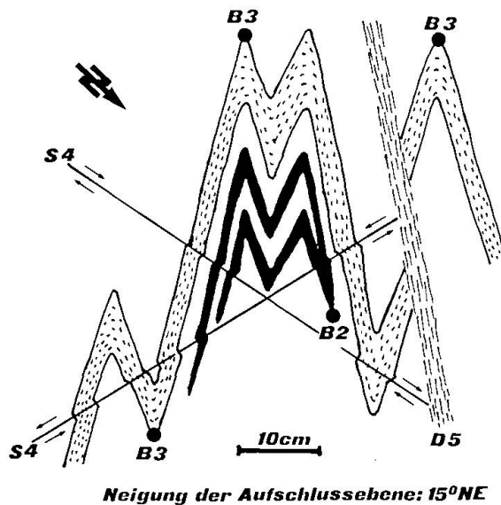
Abb. 6 Schematische Darstellung der strukturellen Entwicklung im Radönt (B3: 35° SW).
