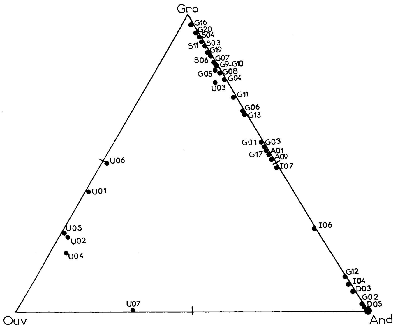
Fig. 2 Localisation dans le diagramme ternaire Ouv-Gro+(Alm+Pyr+Spe)-And des échantillons de grenats caliques étudiés en Raman. Le pôle And regroupe les échantillons D01, D02, D04, G14 et G18.
