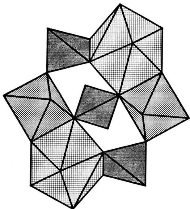
Fig. 1 c) Détail de la configuration des polyèdres dans la structure grenat. Dans la nature X, Y et Z sont occupés par les cations X = Mg^{2+}, Fe^{2+}, Mn^{2+}, Ca^{2+}, (Zn^{2+}), (Na^+) ou (REE) dans les dodécaèdres; Y = Al^{3+}, Cr^{3+}, Fe^{3+}, Ti^{4+}, Ti^{3+}, V^{2+}, Fe^{2+}, (Zr^{2+}) ou (Sn^{4+}) dans les octaèdres; Z = Si^{4+}, Fe^{3+}, (P^{5+}), (Ti^{4+}) ou (Al^{3+}) dans les tétraèdres. Les parenthèses indiquent des substitutions rares ou peu sûres. Chaque oxygène est lié à la fois aux trois types de polyèdres (1T, 1O et 2D) qui partagent entre eux des arêtes ou des sommets mais pas de faces. Ces dessins ont utilisé le logiciel «ATOMS» d'Eric Dowty de SHAPE SOFTWARE (R).
