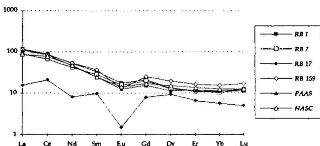
Abb. 1 Vergleich: Lithologien der Silvrettedecke (RB 1 = Feldspatknötengneis, RB 7 = Biotitplagioklasgneis; RB 17 = Muskovitplagioklasgneis; RB 159 = Augengneis Typ Tschuggen) mit postarchaischen Metasedimenten aus Amerika (NASC = North American Shale Composite) und Australien (PAAS = Post Archean Australian Shist) (TAYLOR und McLENNAN, 1985).
