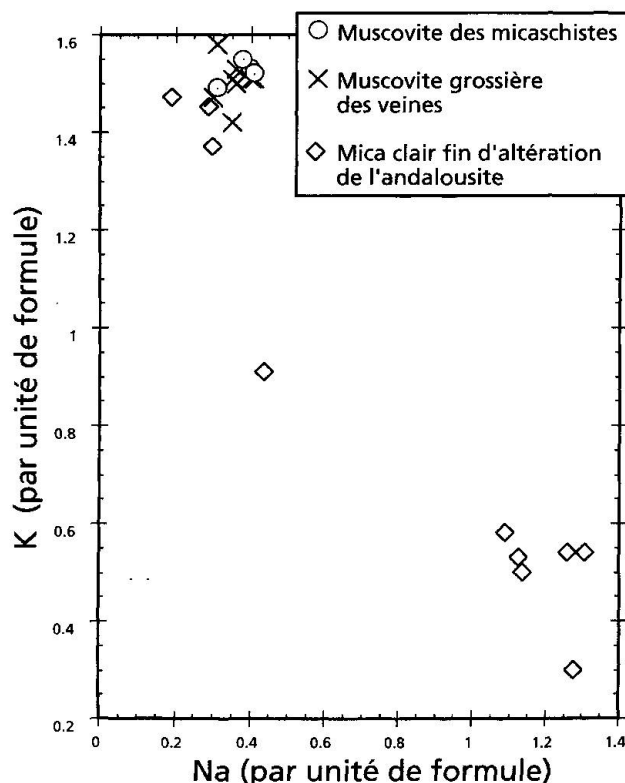
Fig. 2 Rapports Na/K (atomes par unité de formule, normalisation sur 22 oxygènes) dans différentes générations de mica clairs (analyses ponctuelles à la microsonde électronique).
