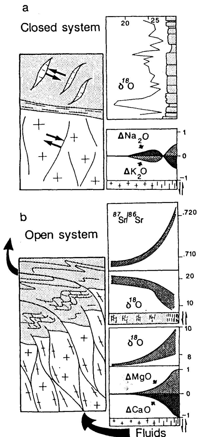
Fig. 1 Les relations socle-couverture: schéma de l'évolution des transferts de matière, des circulations fluides et de la déformation progressive dans la croûte supérieure. (a) Initiation des instabilités mécaniques dans le socle et la couverture. (b) Propagation de la déformation et création d'un réseau anastomose de discontinuités structurales permettant la circulation des fluides entre le socle et la couverture.
